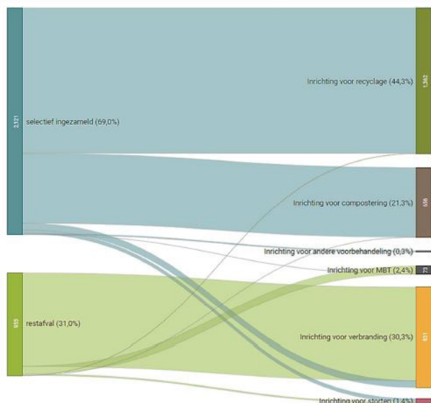
Figuur 2: Stroomdiagram met aanduiding van de inrichting voor verwerking van het selectief ingezameld huishoudelijk afval en het restafval in het Vlaamse Gewest in 2017 (hoeveelheden in kton). MBT= mechanisch-biologische scheidingsinstallatie
